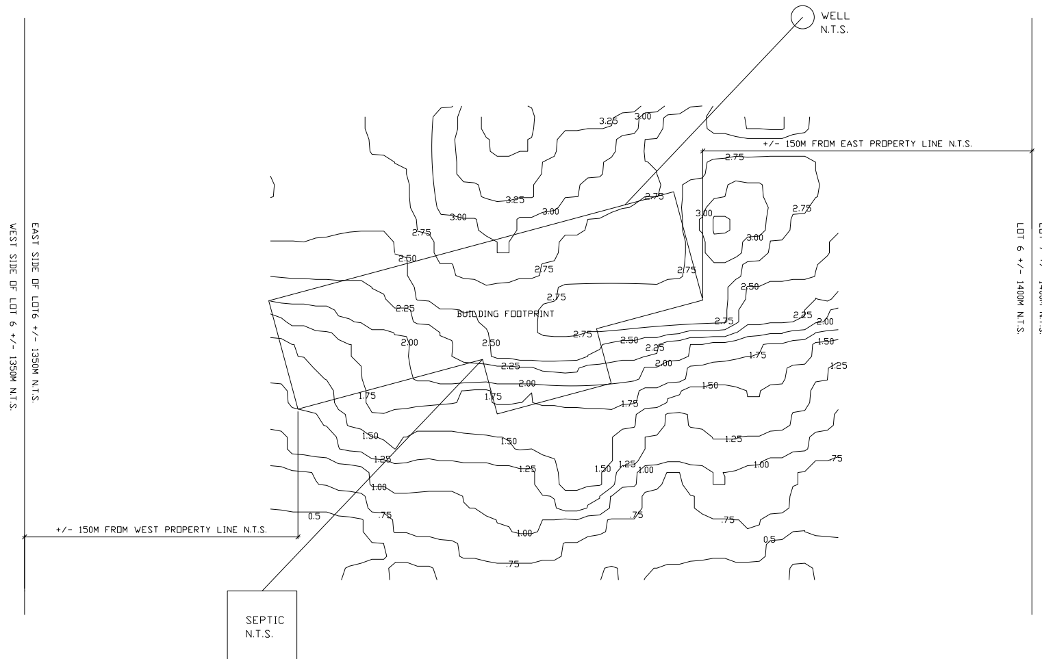
1 SITE PLAN 01 1:100
